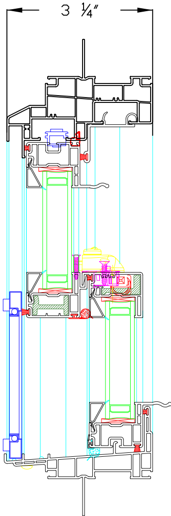
Section A-A
