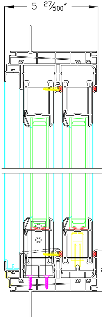
Section A-A
